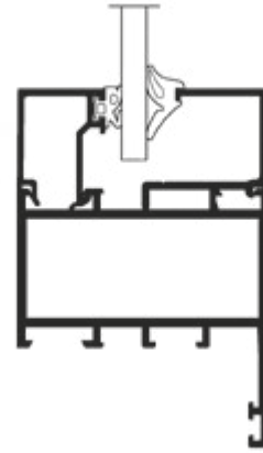
MITTIGE VERGLASUNG
