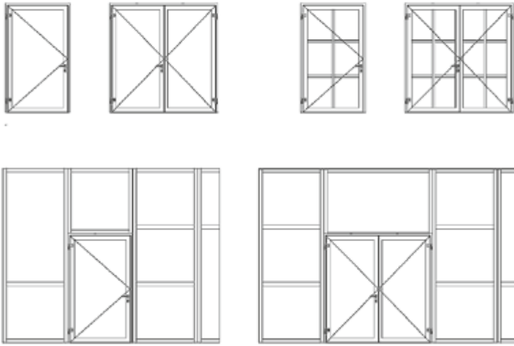
ÖFFNUNGSARTEN
