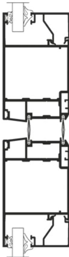
PENDELSTÜLP
