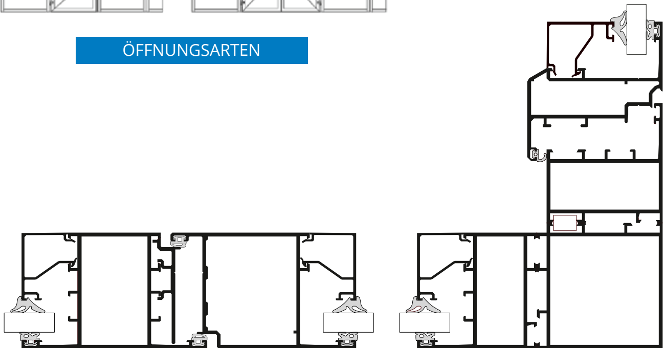
BEISPIELSCHNITT
